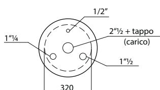
particolare boccaporto
